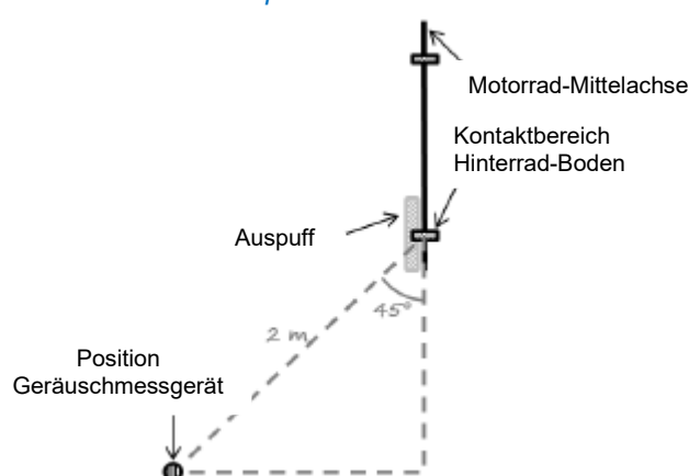
Solomotorrad – Auspuff links - Draufsicht
