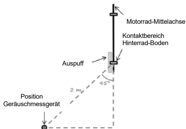
Solomotorrad – Auspuff links - Draufsicht
